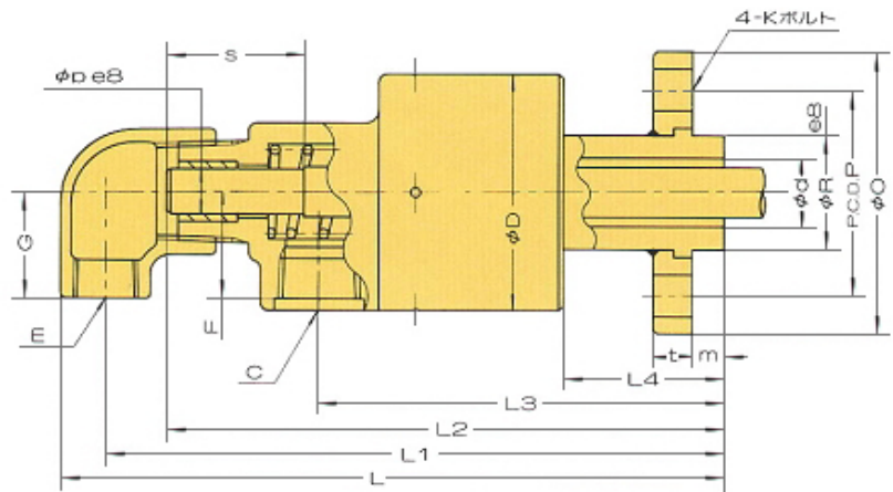
尺寸表 RXE 6100, RXH 6100 复式内管旋转法兰安装式
