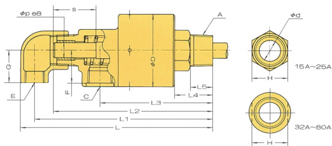
尺寸表 RXE 5000, RXH 5000 复式内管旋转螺纹安装式
